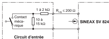
Fig. 3. Câblage des contacts.
