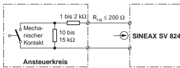
Bild 3. Kontaktbeschaltung.
