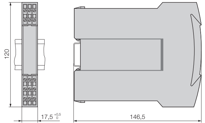
Fig. 14. SINEAX SV 824 en boîtier S17 encliqueté sur rail symétrique «en chapeau» (35 × 15 mm ou 35 × 7,5 mm selon EN 50 022).
